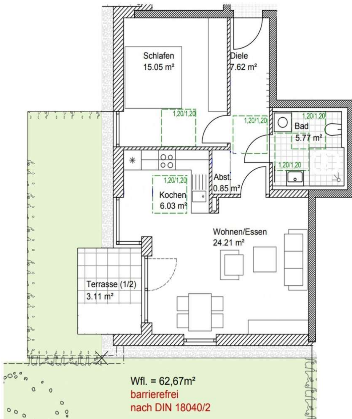
Grundriss
